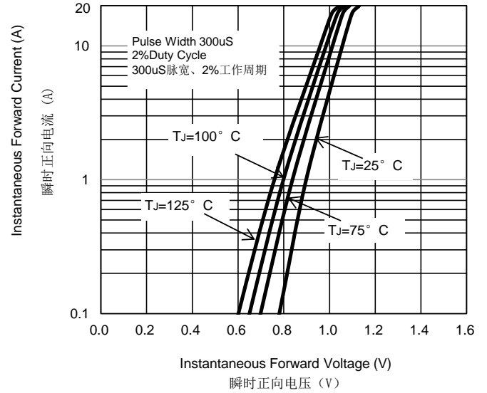
图4 典型的正向特性
