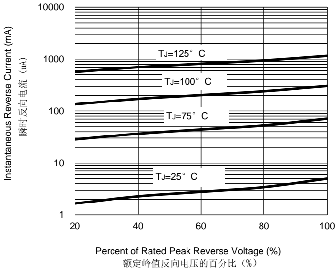
图3 典型的反向特性
